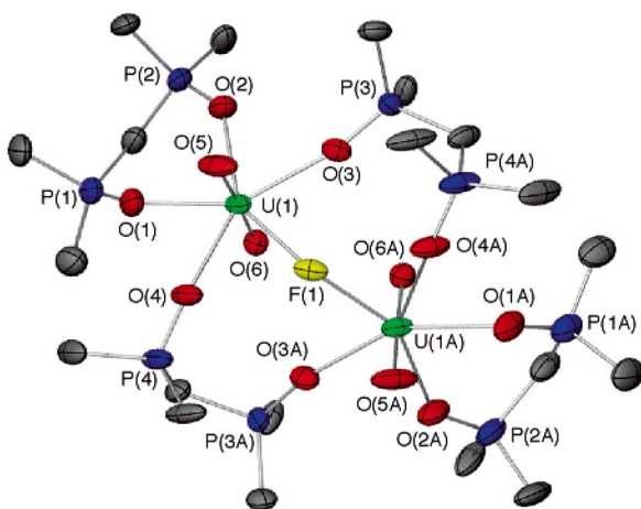
Рис. 7. Молекулярное строение димерного комплексного катиона [(UO_2(dppmo)_2)_2(\mu-F)]^{3+} в структуре [(UO_2(dppmo)_2)_2(\mu-F)][BF_4]_3 [16]
