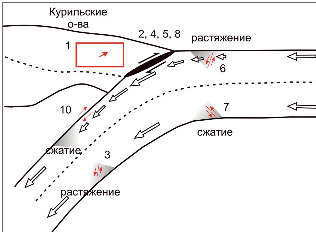
Рис. 4. Модель субдукции и сеймотектонического процесса для Курильской островной дуги. Номер землетрясения на рисунке соответствует порядковому номеру, приведенному в табл. 1
