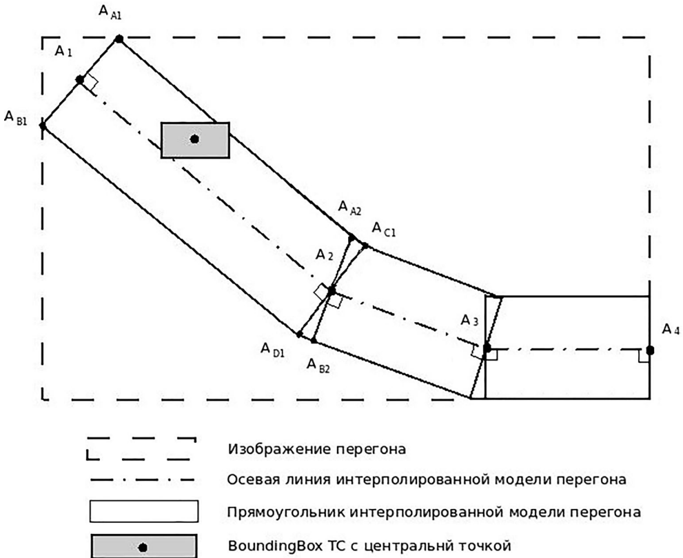
Рис. 4. Направление трафика, определяемое путем нахождения центральной точки гипотенузы и ее положения по отношению к центральной линии интерполированной модели пролетов
