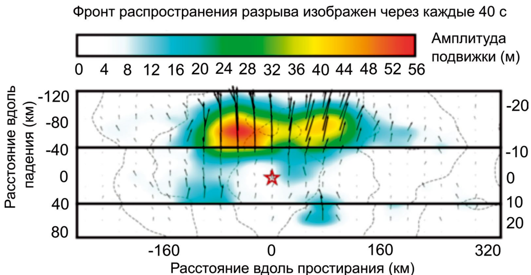
Рис. 3. Распределение вектора подвижки на плоскости разрыва 11 марта 2011 г. в 5:46 в Тохоку (Япония). Эпицентр землетрясения располагался в точке с координатами 38,297° с. ш., 142,373° в. д. Моментная магнитуда составила Mw 9,1, угол простирания (Str) – 198,0°, угол падения (Dip) – 15,0° [19]
