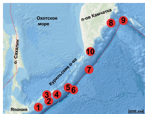
Рис. 2. Землетрясения в районе Курило-Камчатской островной дуги с магнитудой M \geq 7,0 (1–10), для которых доступны данные о распределении вектора подвижки на разрыве (finite fault) [17]
