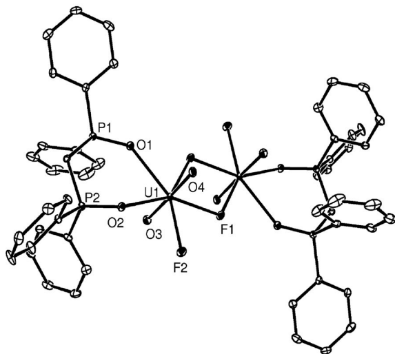
Рис. 5. Молекулярное строение димерного комплекса [UO_2(\mu-F)(F)(DPPMO_2)]_2 в структуре [UO_2(\mu-F)(F)(DPPMO_2)]_2 \cdot 2MeOH [15]
