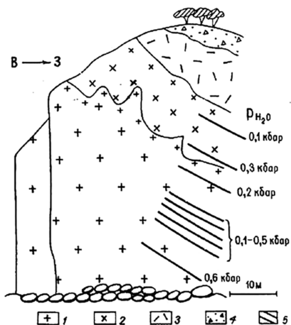
Рис. 4. Вертикальный разрез прикровлевой части Бринеровского массива по одной из расселин перпендикулярно линии берега моря: 1 — турмалиновые граниты, 2 — гранофировые гранодиориты, 3 — риолит-дациты кровли, 4 — делювий, 5 — изолинии P_{H_2O} согласно составу гранофилов. Серия частых линий 0,1–0,5 кбар — зона ритмичного гранофир-аплитового расслоения в турмалиновых гранитах [1]
