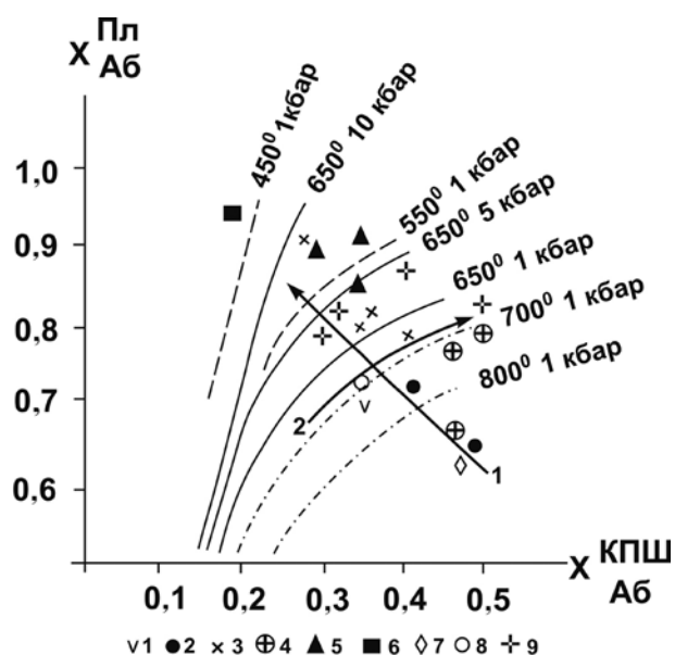
Рис. 1. Распределение натрия между сосуществующими плагиоклазами и КПШ: 1–8 – ассоциация плагиоклаза с антипертитовым КПШ: 1 – в диоритах, 2 – гранодиоритовых включениях, 3 – гранитах центральных частей массивов, 4 – гранитах приконтактных фаций, 5 – пегматитах и аплитно-пегматитовых дайках, 6 – метасоматически измененных гранитах, 7 – гранодиоритах, 8 – малоглубинных гранитах; 9 – ассоциация внешних зон плагиоклазов с самостоятельными кристаллами КПШ. Штрих-пунктирные линии проведены по данным работы [14], сплошные и пунктирные – по данным работы [16]; линии 1 и 2 – изменение P_{H_2O} в процессе кристаллизации более и менее глубоких интрузивов соответственно
