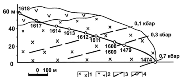
Рис. 3. Схематический разрез Бринеровского интрузива вдоль русла кл. Быстрый. 1 — гранодиориты, 2 — вмещающие эффузивы, 3 — изолинии P_{H_2O} согласно составу гранофилов, 4 — места отбора образцов
